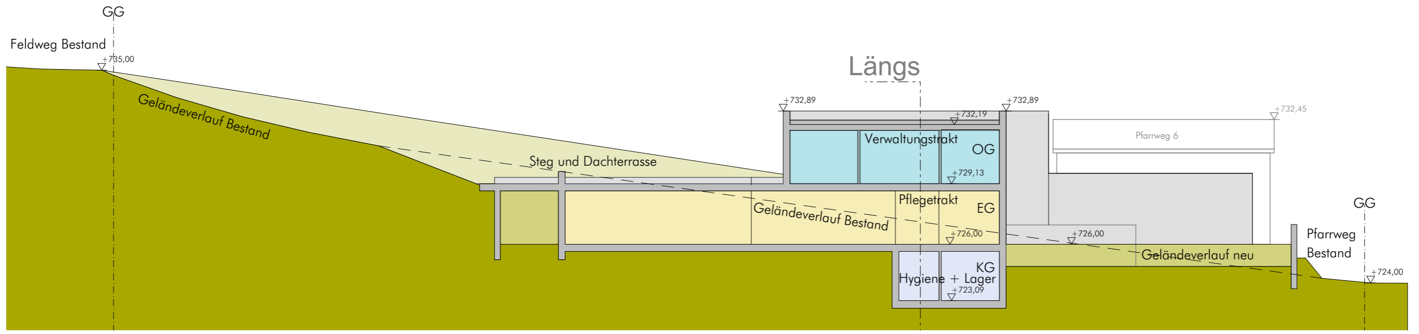
Schnitt A
