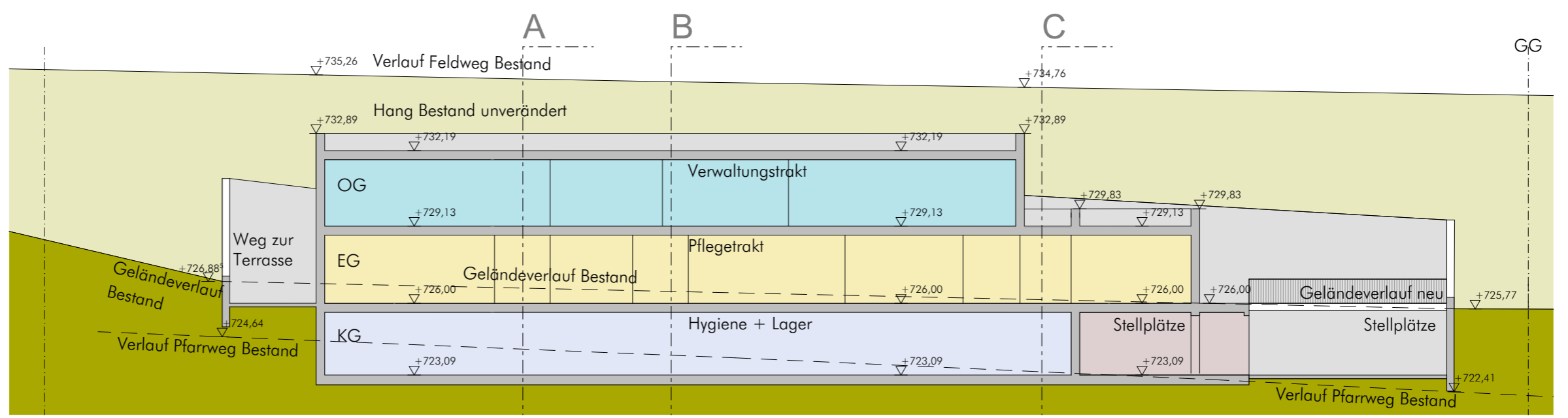
Schnitt Längs
