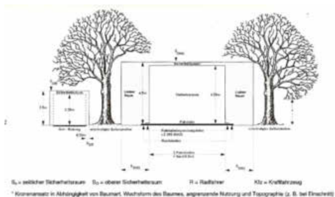
Abb. 2: Beispielhafte Darstellung des Lichter Raumes in Anlehnung an RAS-Q für anbaufreie Straßen
