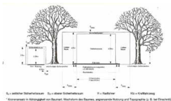
Abb. 2: Beispielhafte Darstellung des Lichter Raumes in Anlehnung an RAS-Q für anbaufreie Straßen
